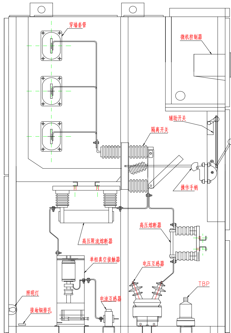
图 2 消弧消谐及过电压保护综合装置结构图(侧视)
