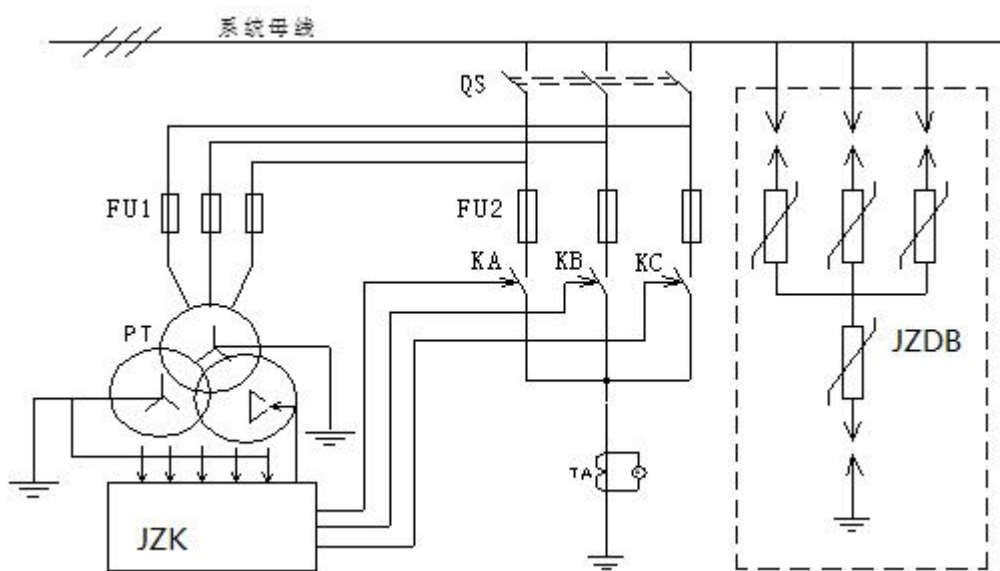
图 1 消弧消谐及过电压保护装置电气原理图
